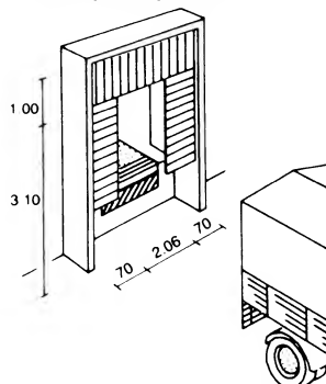
11 Rubber segment door seal
